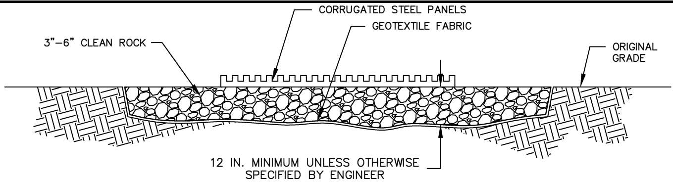
SECTION A-A
